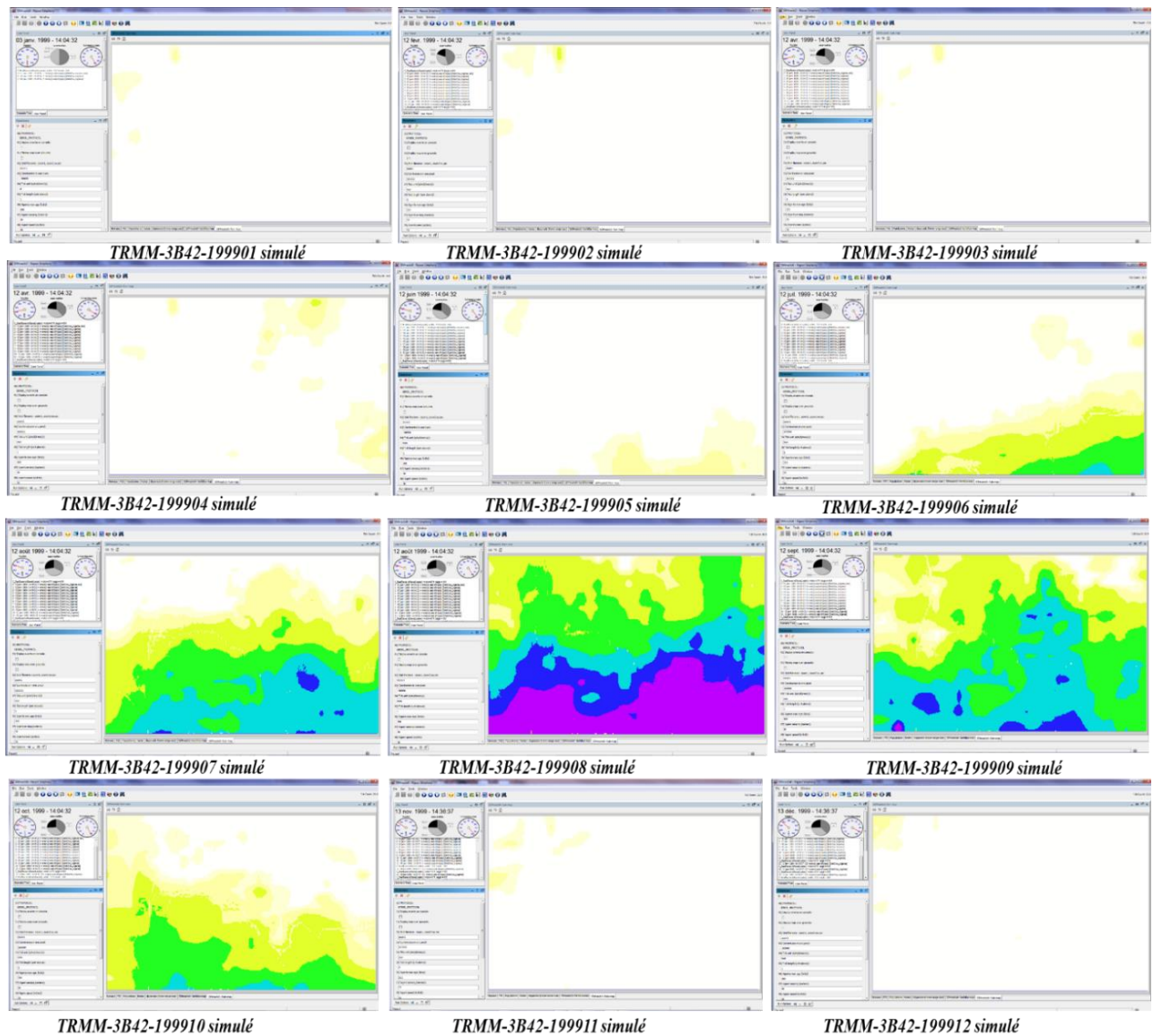
Figure 10 : Simulation de la pluviométrie de l'année 1999 (Sall, 2016)
